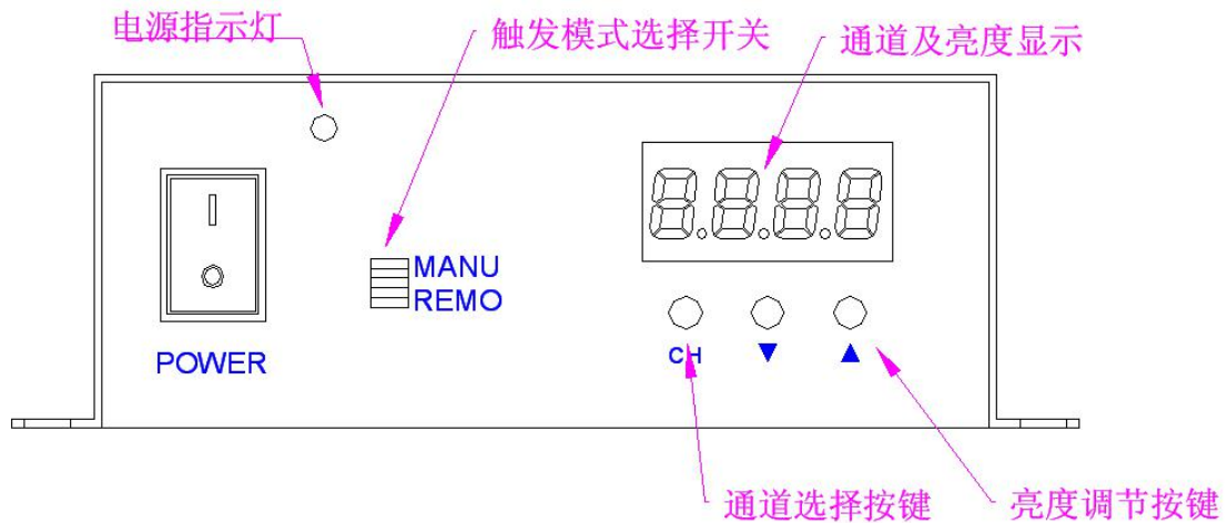
图 1 前面板各部件功能示意图
